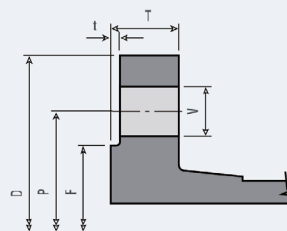
PN16 FLANGES
